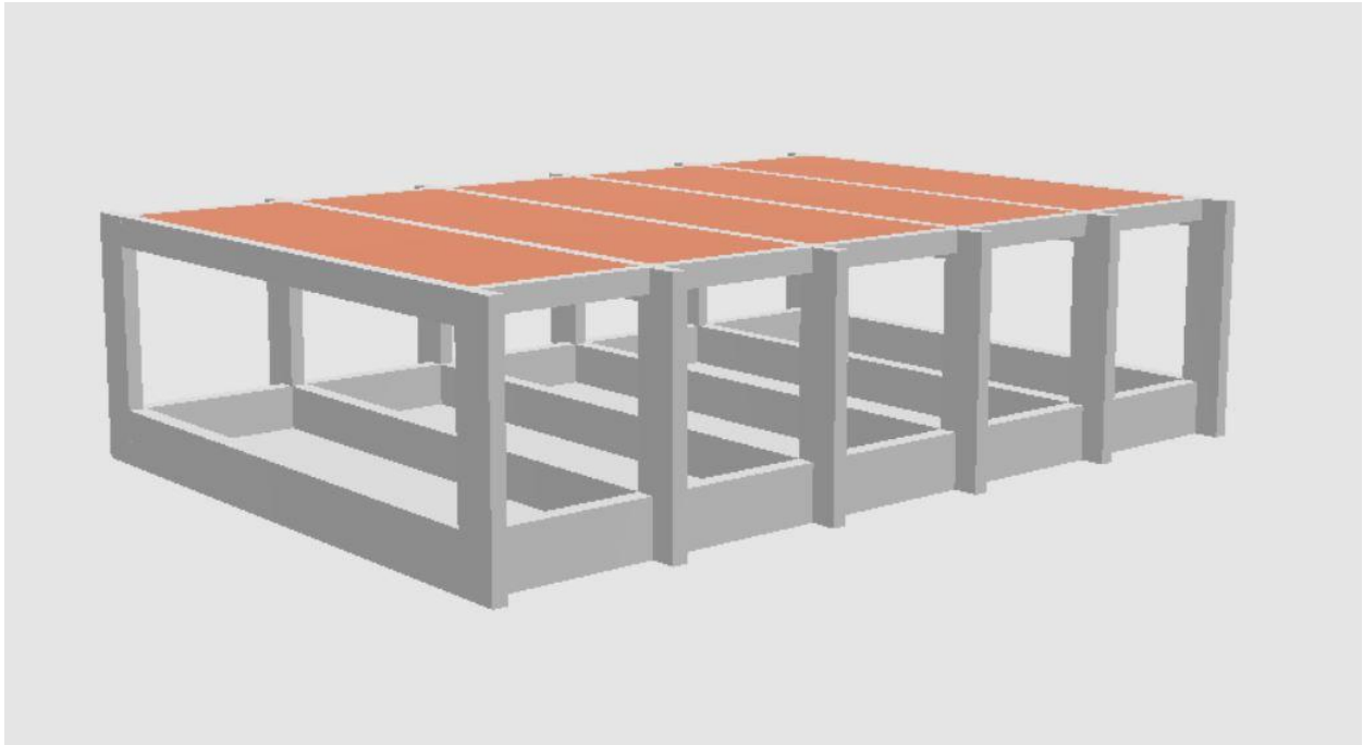
Figura 1: Vista Assonometrica Anteriore Generale della Struttura - “Corpo H”
