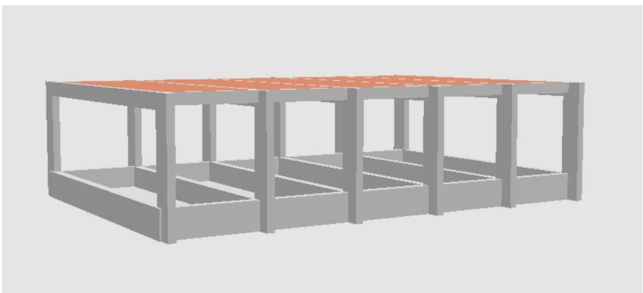
Figura 2: Vista Assonometrica Posteriore Generale della Struttura - “Corpo H”
