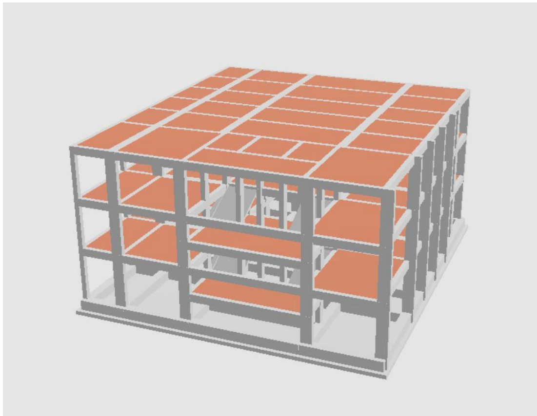
Figura 2: Vista Assonometrica Posteriore Generale della Struttura - “Corpo D”
