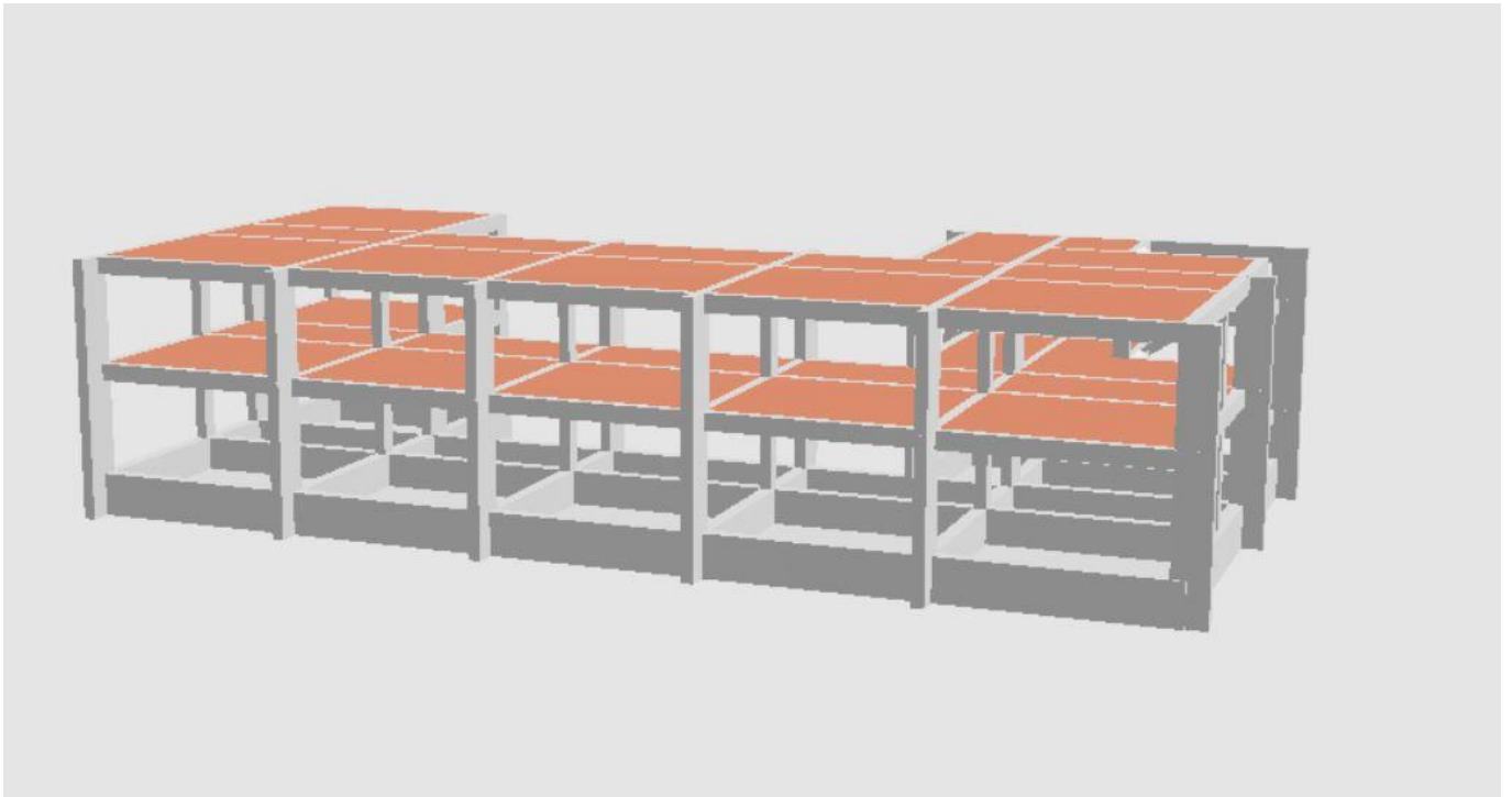
Figura 1: Vista Assonometrica Anteriore Generale della Struttura - “Corpo C”
