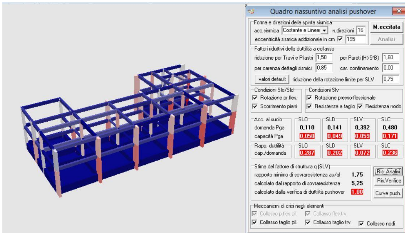
Figura 3: Valutazione Struttura mediante analisi pushover
