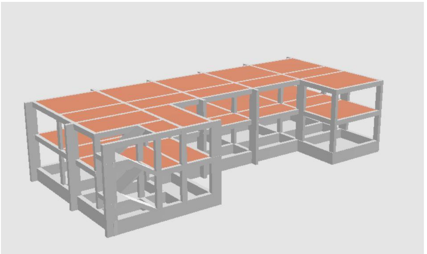
Figura 2: Vista Assonometrica Posteriore Generale della Struttura - “Corpo C”
