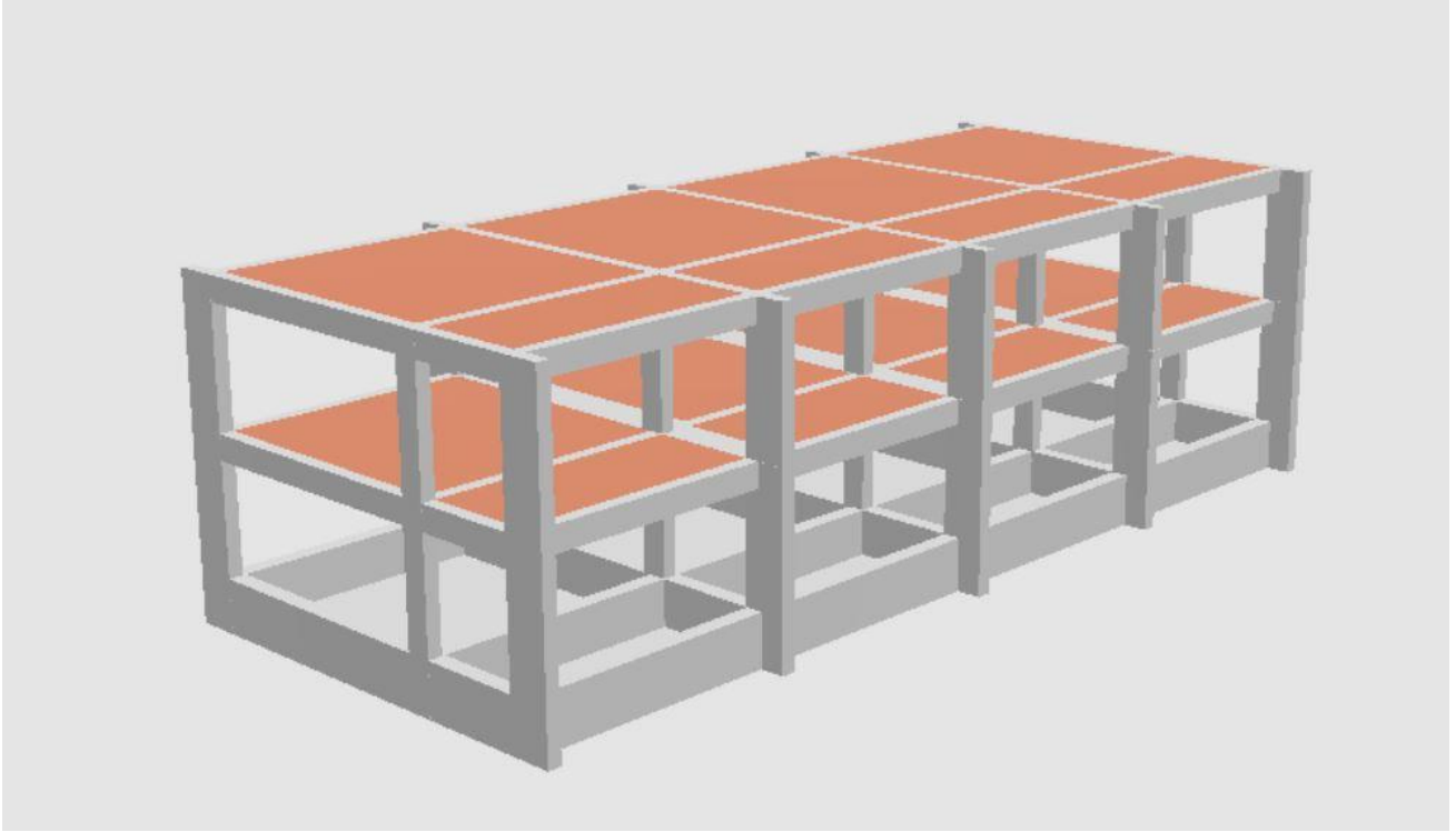
Figura 1: Vista Assonometrica Anteriore Generale della Struttura - “Corpo B”
