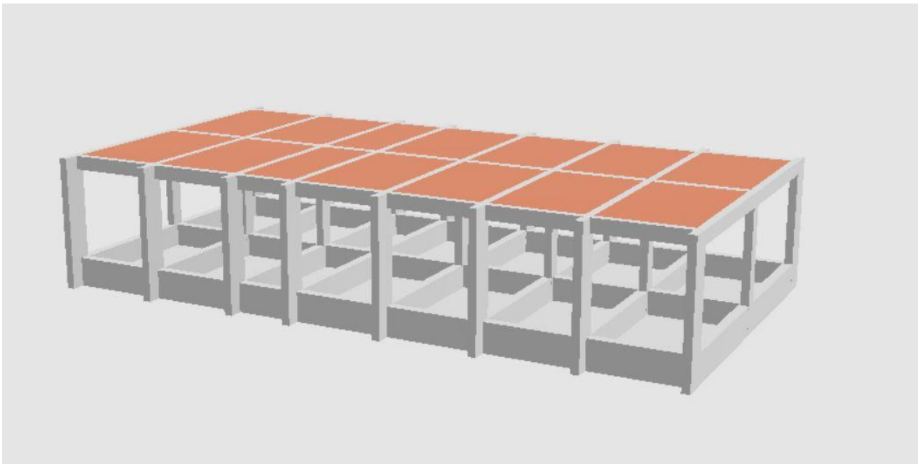
Figura 1: Vista Assonometrica Anteriore Generale della Struttura - “Corpo A”
